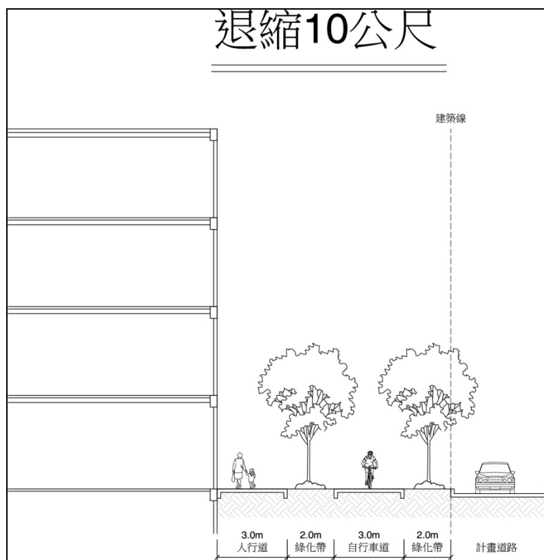
附圖 2-1 自道路境界線退縮 10 公尺之退縮空間斷面示意圖
