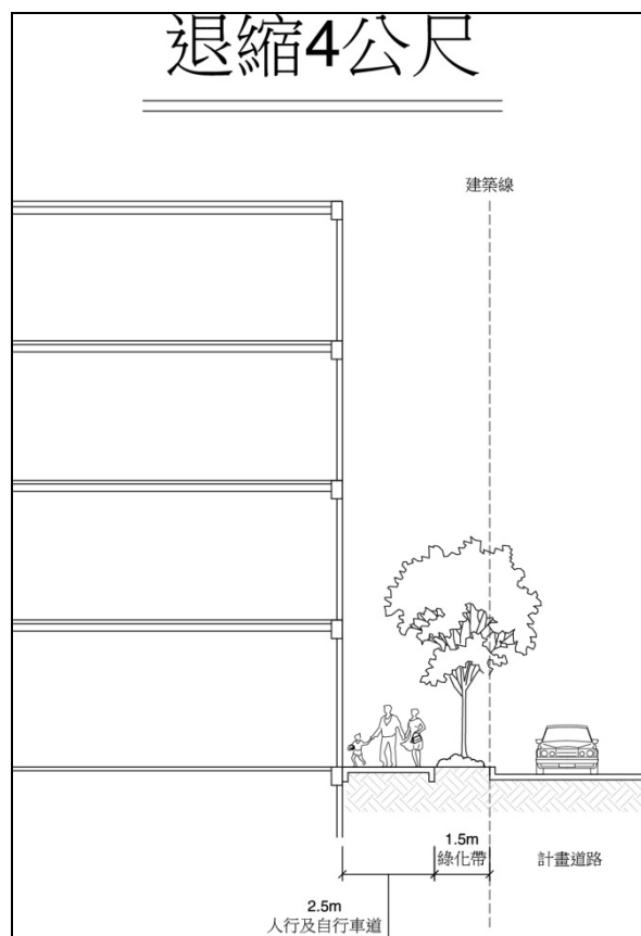
附圖 2-3 自道路境界線退縮 4 公尺之退縮空間斷面示意圖
